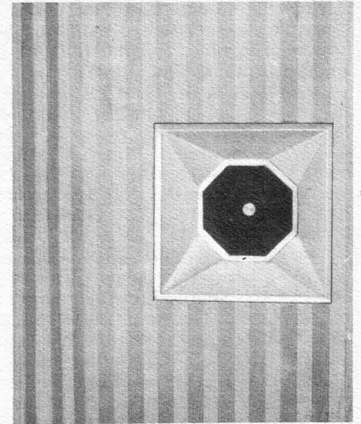
Abb. 5. Ein in eine 15-cm-Wand eingefetzter Einbau-Kasten mit montiertem Dynamischen. (Die 4 Ecken sind hier noch mit dreieckigen Holzteilen ausgefüllert, was zwar empfehlenswert, aber nicht unbedingt nötig ist.) Sämtl. Aufnahmen vom Verfasser
