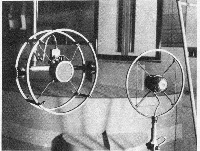
Zwei der bei der englischen Sendegesellschaft nunmehr allgemein eingeführten Bändchen-Mikrophone. Photo B. B. C. London.
