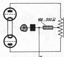
Abb. 4. Schutzwiderstand gegen Pfeifen.
