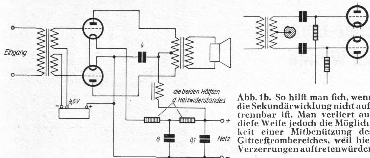
O b e n Abb. 1a. Eine gewöhnliche Gegentaktendstufe für Gleichstromnetzanschluß mit direkt geheizten Röhren und Gitter-batterie.
