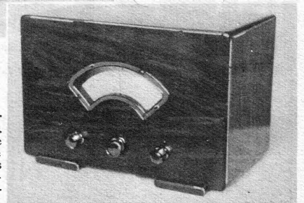
Der Vorkämpfer-Superhet für Allstrom (FUNKSCHAU-Baupl. Nr. 340) in vorbildlicher Weise aufgebaut und mit Gehäuse ausgestattet. „Die Leistung des Gerätes übertrifft meine Erwartungen“, schreibt der Verfasser. Photo Karl Friedrich.
