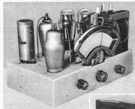
Ebenfalls ein Vorkämpfer-Superhet fein fauberlich in einem Gehäuse. Aufnahme Arthur Bein.
